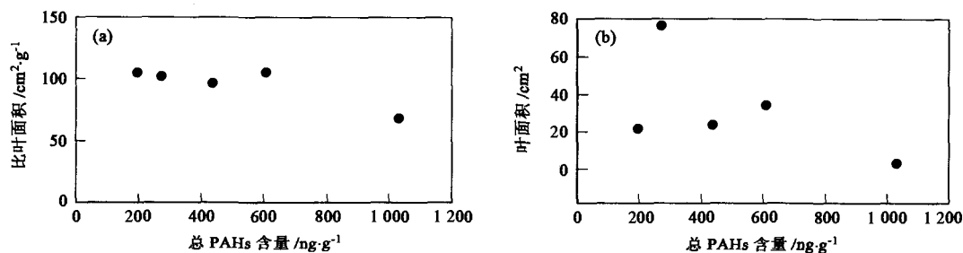
图 5 PAHs 含量与比叶面积、叶面积的关系
