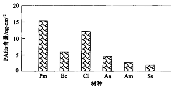
图 6 6 种植物叶片单位叶面积上的 \sum PAHs 含量
