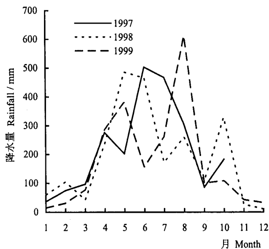
图 1 鼎湖山马尾松林 1997~1999 年林外降水月分配格局
