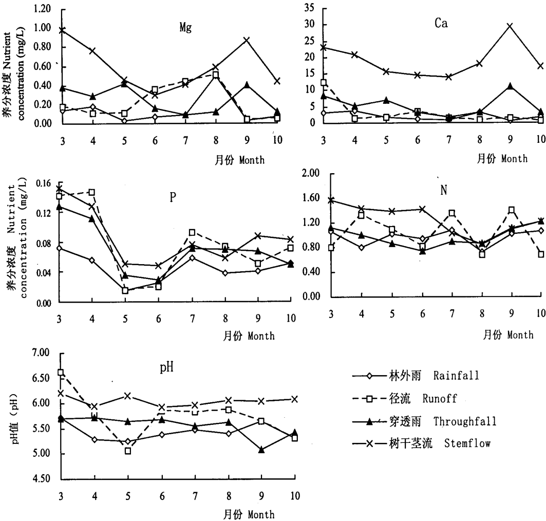
图 2 pH 值、养分浓度的月变化 Fig. 2 The monthly rhythm of pH and nutrient concentrations
