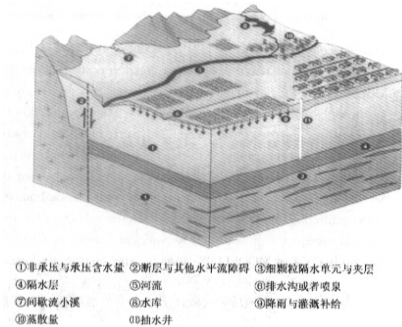
图 1 MODFLOW 可以模拟的地下水含水层系统
