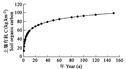
图 1 南亚热带阔叶混交林土壤有机 C 随植被恢复进程的变化曲线 [33]
